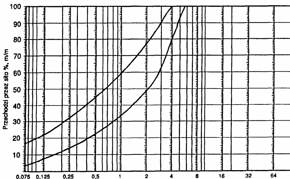
Rys. 1. Krzywa dobrego uziarnienia mieszanki od 0 do 4 mm
